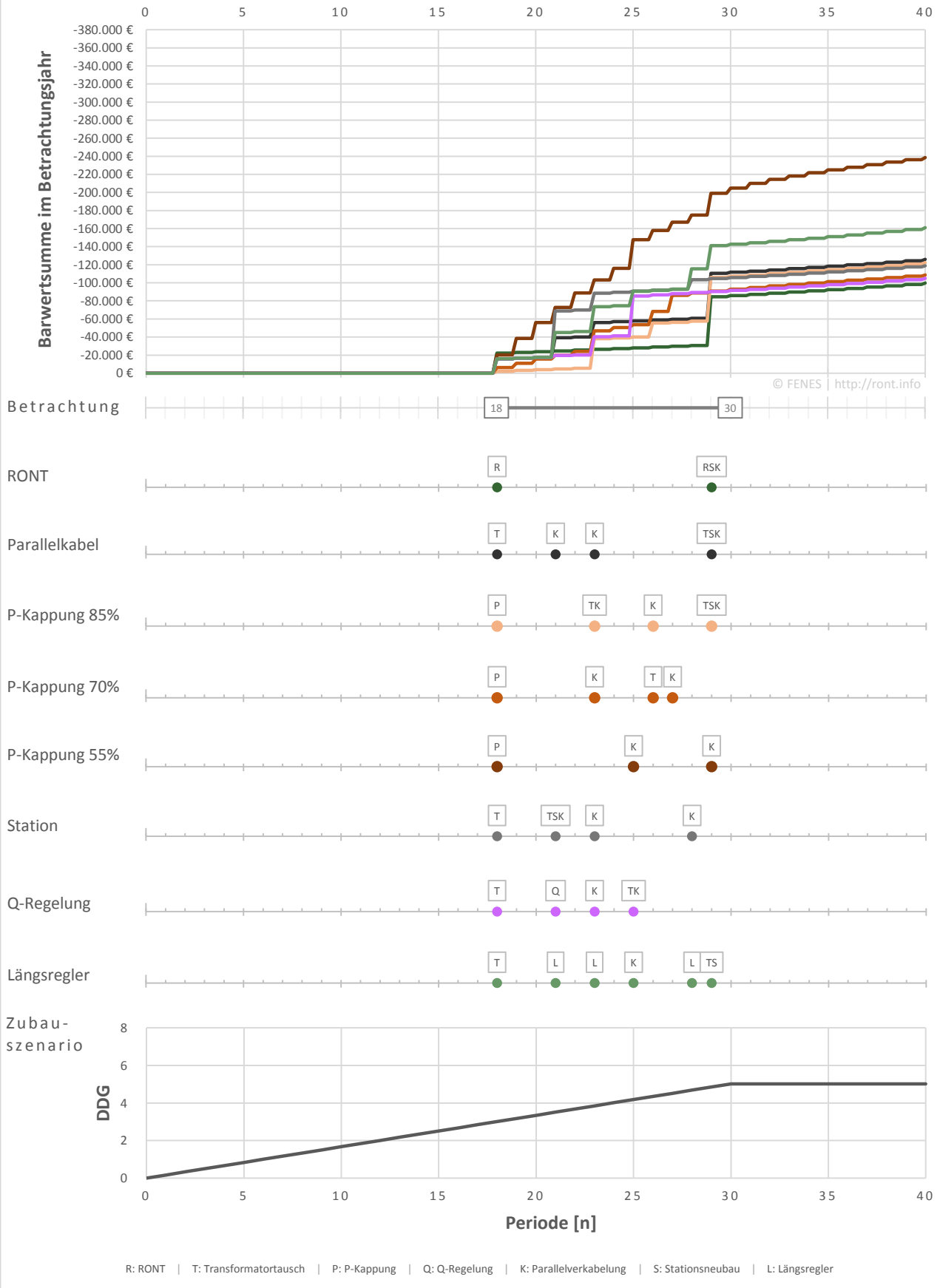
Abbildung 1: Zubau über 40 Jahre auf DDG_{norm} = 75\% , Stranganfang, i = 5\% | r = 1,5\% (FLE1)
