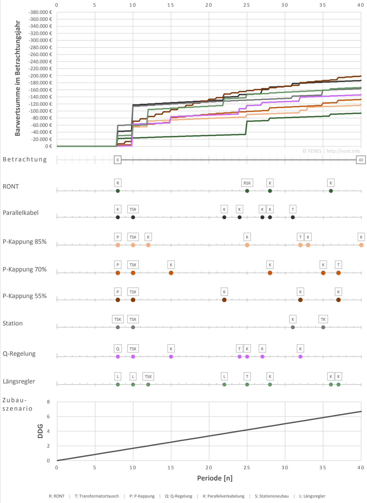
Abbildung 4: Zubau über 40 Jahre auf DDG_{norm} = 100\% , Strangende, i = 5\% \mid r = 1,5\% (FLE1)
