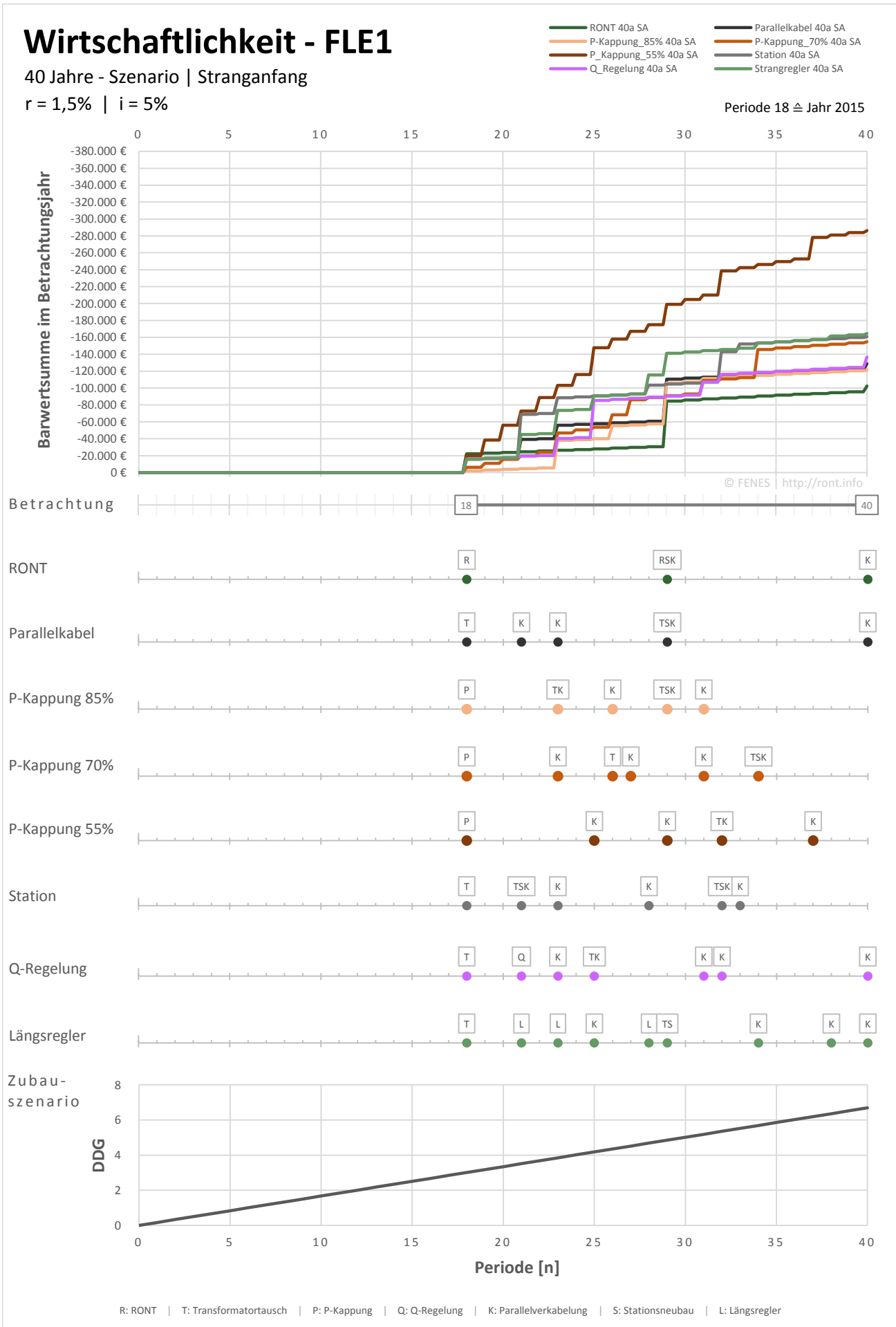
Abbildung 3: Zubau über 40 Jahre auf DDG_{norm} = 100\% , Stranganfang, i = 5\% | r = 1,5\% (FLE1)
