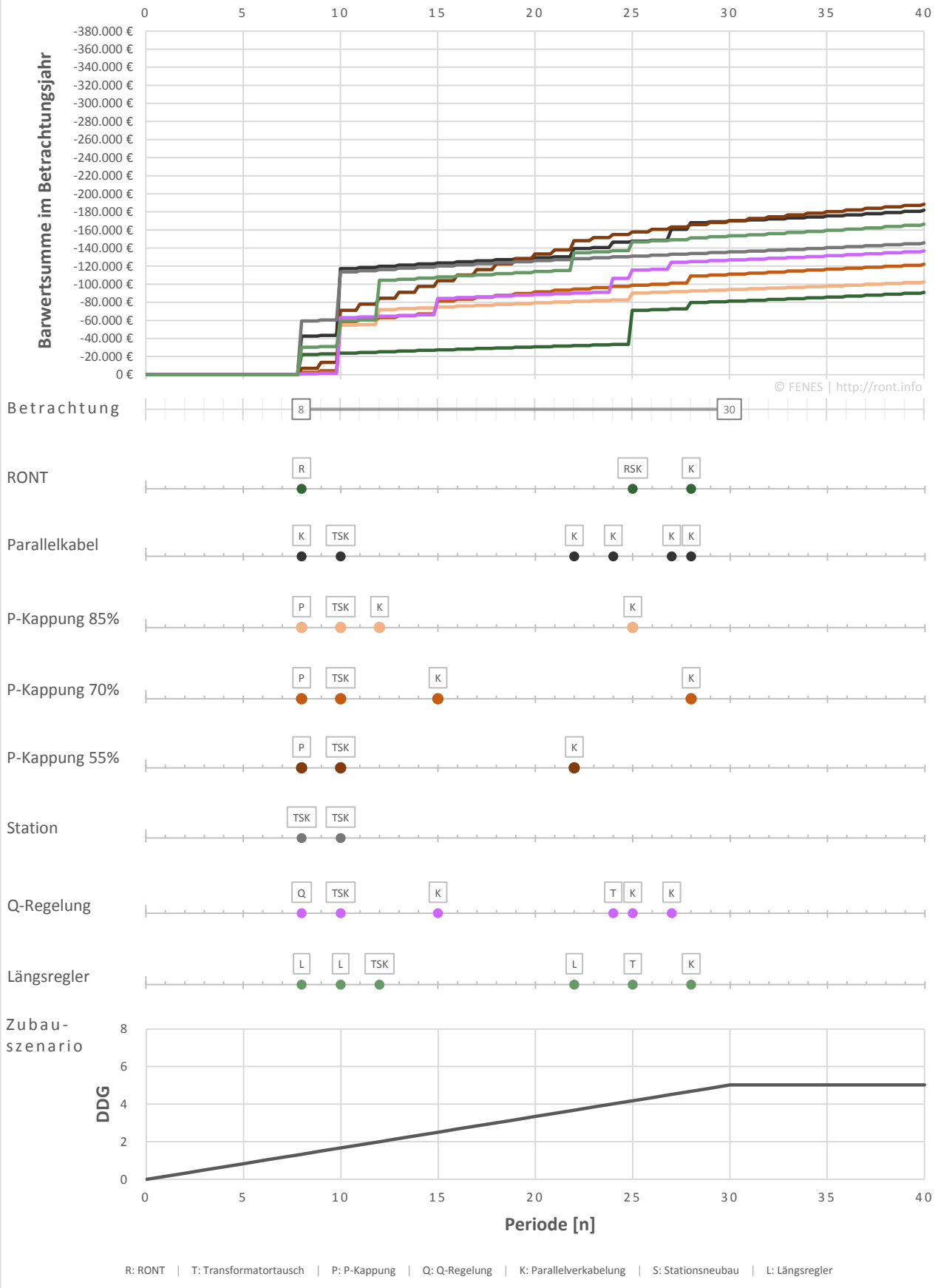
Abbildung 2: Zubau über 40 Jahre auf DDG_{norm} = 75\% , Strangende, i = 5\% | r = 1,5\% (FLE1)
