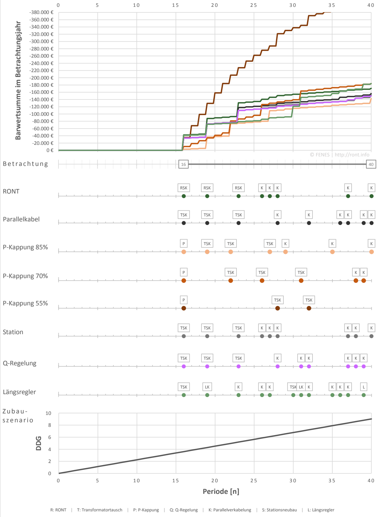
Abbildung 3: Zubau über 40 Jahre auf DDG_{norm} = 100\% , Stranganfang, i = 5\% | r = 1,5\% (FVE1)
