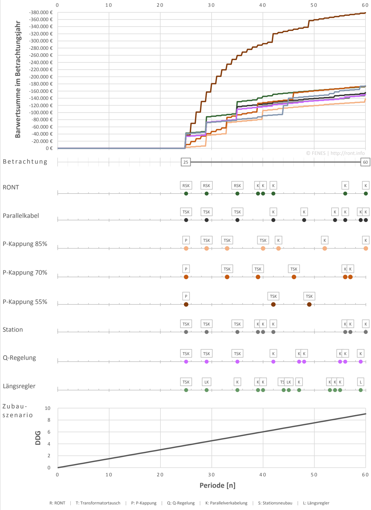
Abbildung 5: Zubau über 40 Jahre auf DDG_{norm} = 100\% , Stranganfang, i = 5\% | r = 1,5\% (FVE1)
