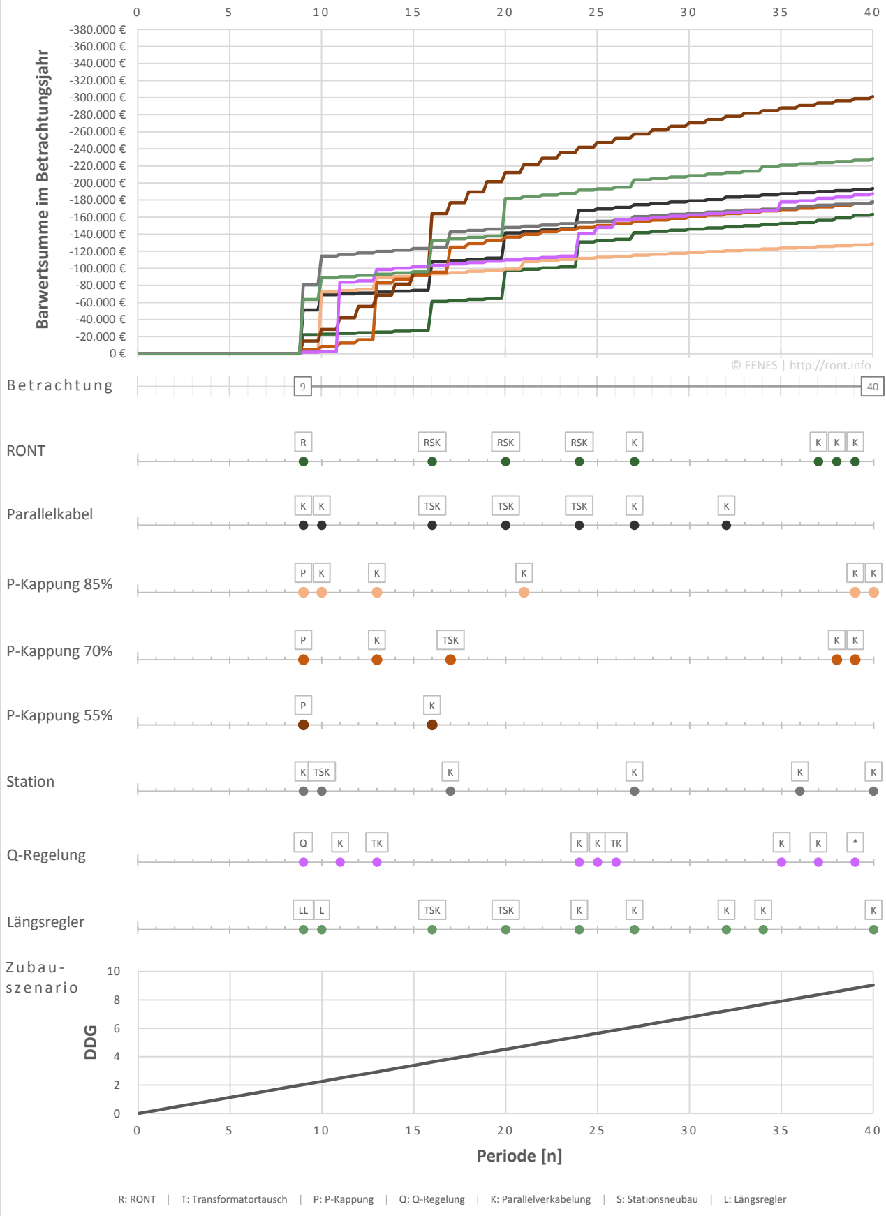
Abbildung 4: Zubau über 40 Jahre auf DDG_{norm} = 100\% , Strangende, i = 5\% | r = 1,5\% (FVE1)
