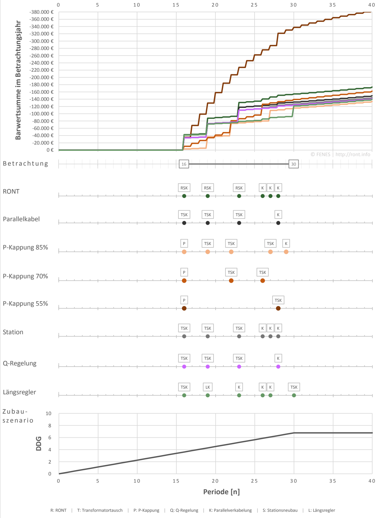
Abbildung 1: Zubau über 40 Jahre auf DDG_{norm} = 75\% , Stranganfang, i = 5\% | r = 1,5\% (FVE1)
