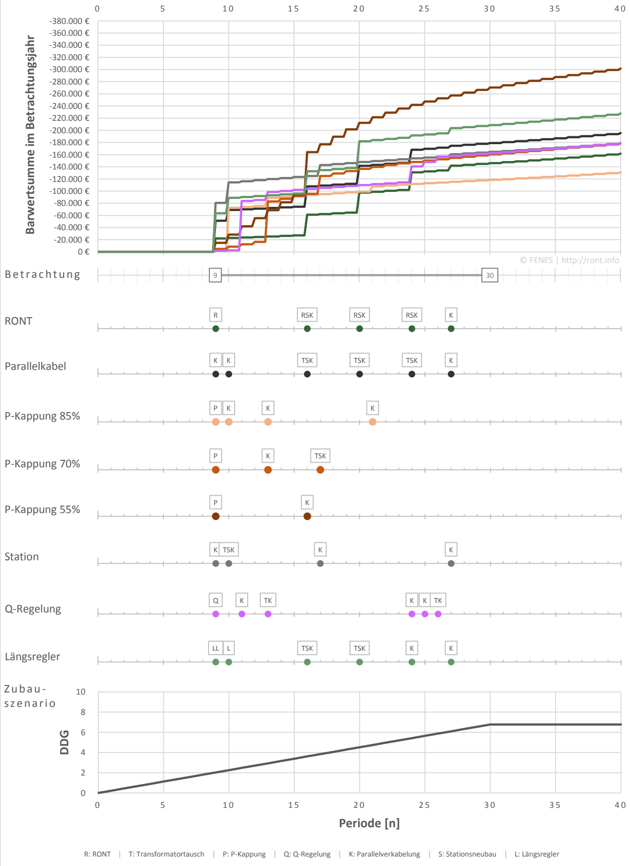
Abbildung 2: Zubau über 40 Jahre auf DDG_{norm} = 75\% , Strangende, i = 5\% | r = 1,5\% (FVE1)
