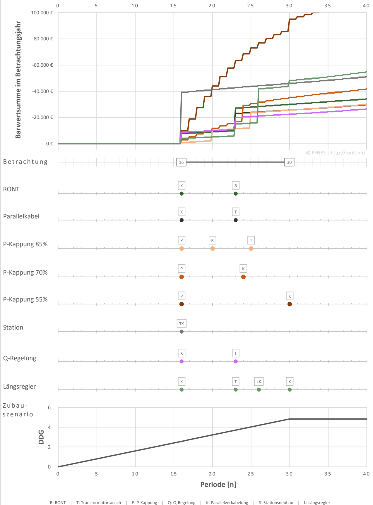
Abbildung 1: Zubau über 40 Jahre auf DDG_{norm} = 75\% , Stranganfang, i = 5\% | r = 1,5\% (KLE1)
