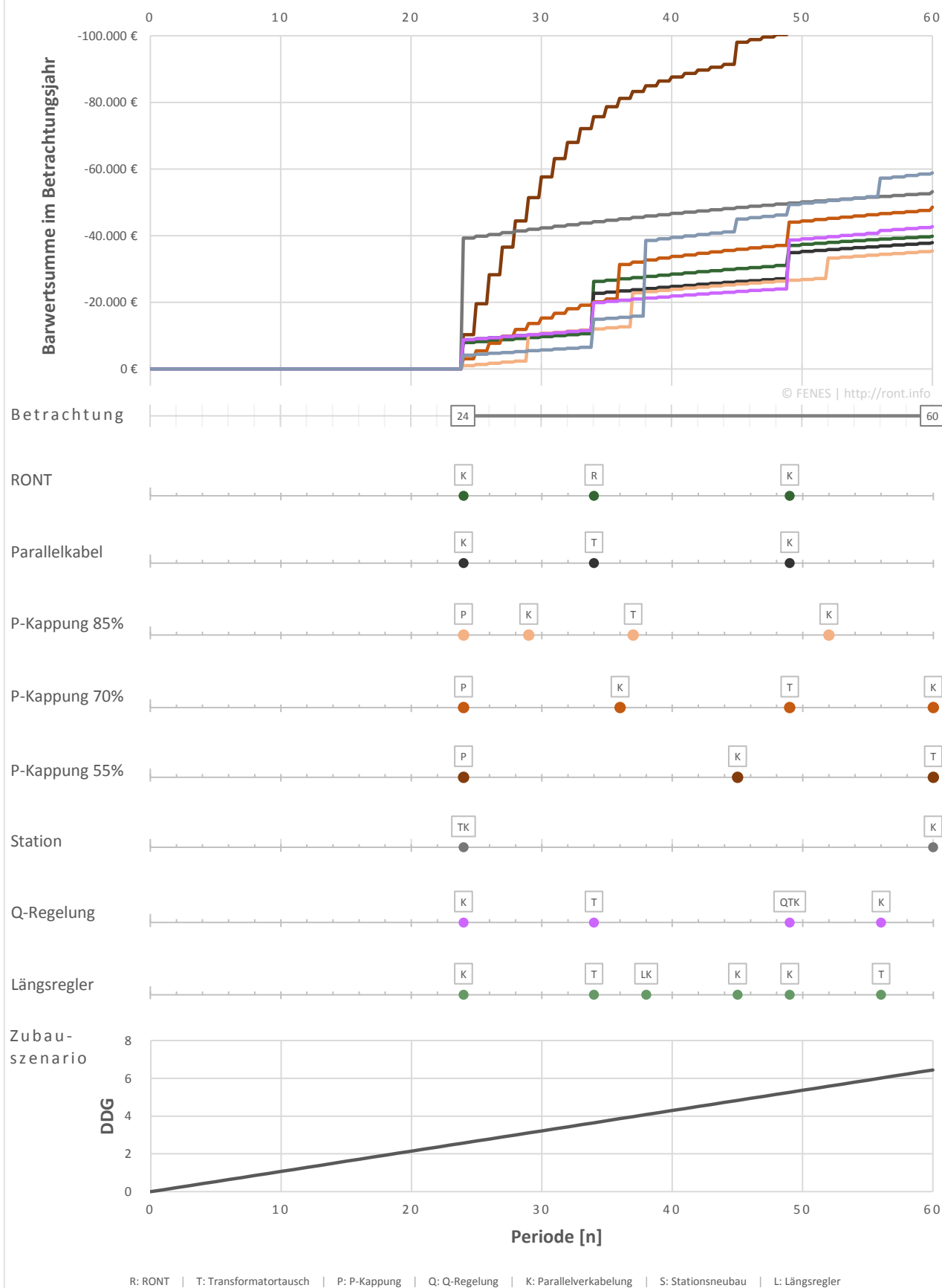
Abbildung 5: Zubau über 40 Jahre auf DDG_{norm} = 100\% , Stranganfang, i = 5\% | r = 1,5\% (KLE1)
