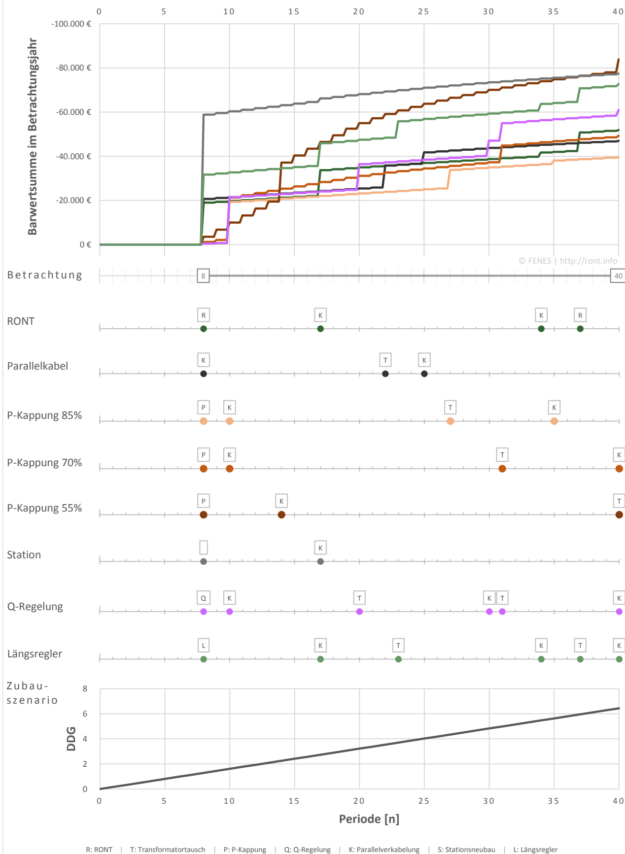
Abbildung 4: Zubau über 40 Jahre auf DDG_{norm} = 100\% , Strangende, i = 5\% | r = 1,5\% (KLE1)
