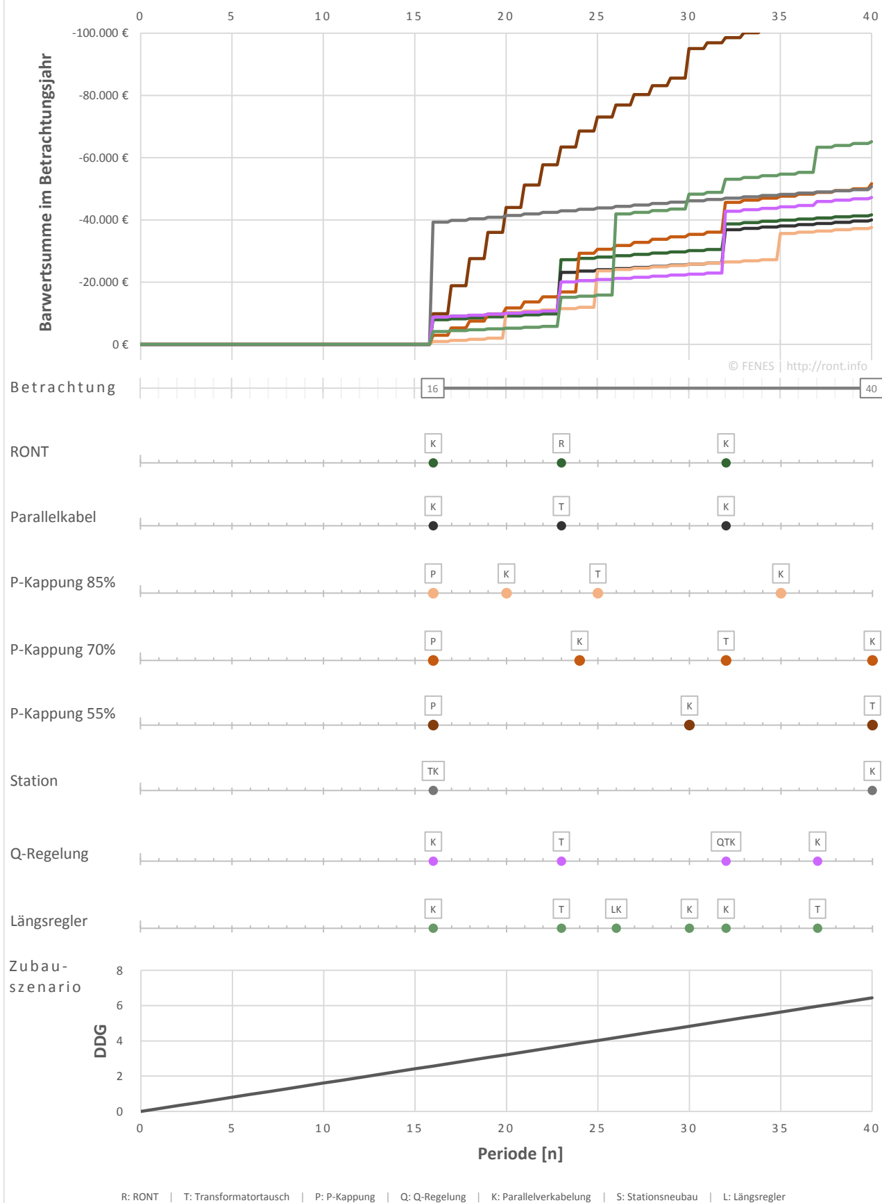
Abbildung 3: Zubau über 40 Jahre auf DDG_{norm} = 100\% , Stranganfang, i = 5\% | r = 1,5\% (KLE1)
