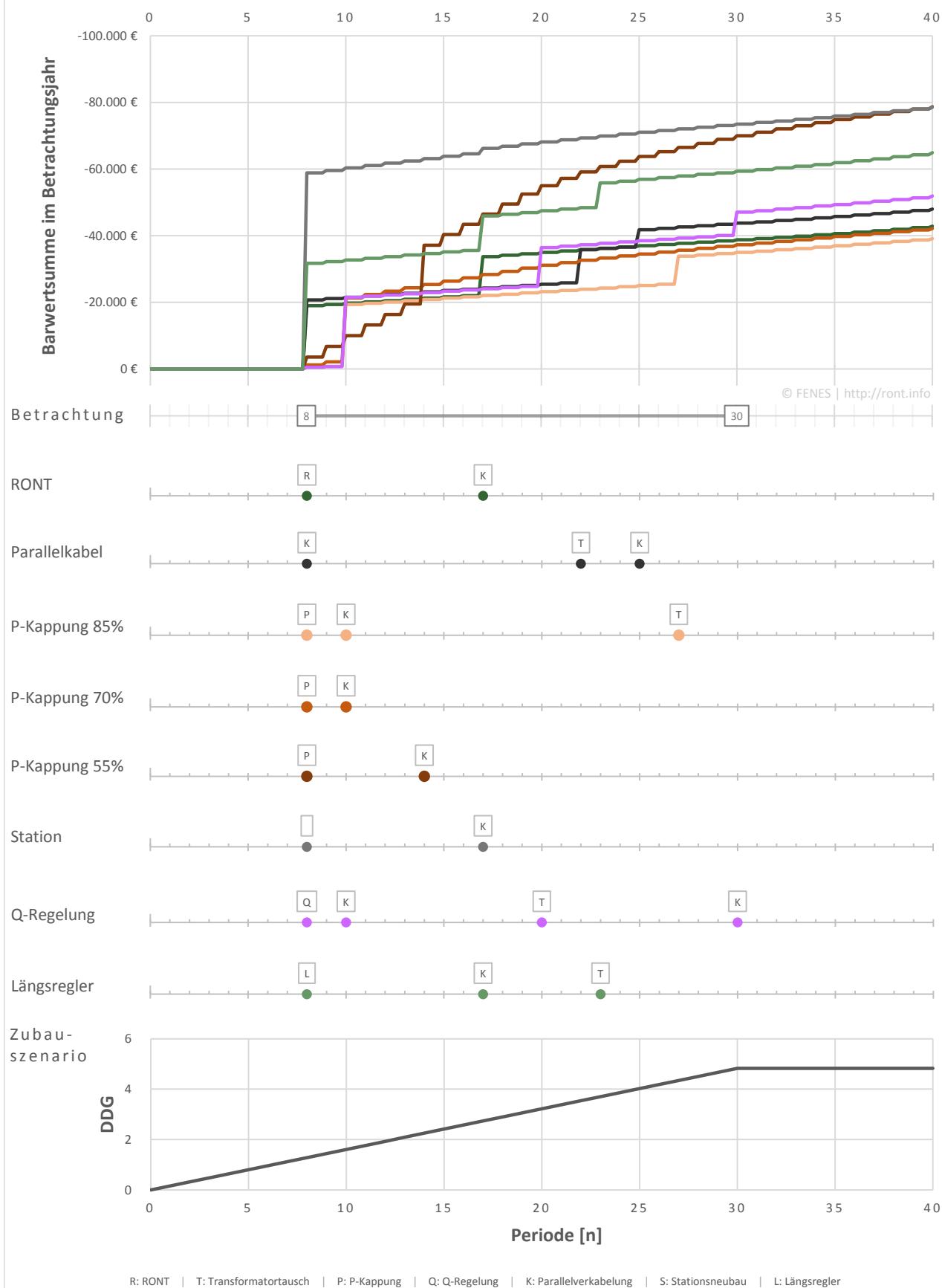
Abbildung 2: Zubau über 40 Jahre auf DDG_{norm} = 75\% , Strangende, i = 5\% | r = 1,5\% (KLE1)
