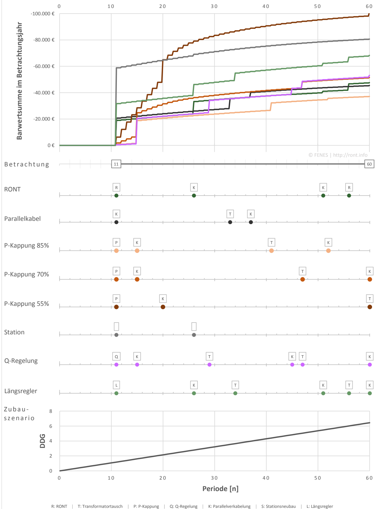
Abbildung 6: Zubau über 40 Jahre auf DDG_{norm} = 100\% , Strangende, i = 5\% | r = 1,5\% (KLE1)
