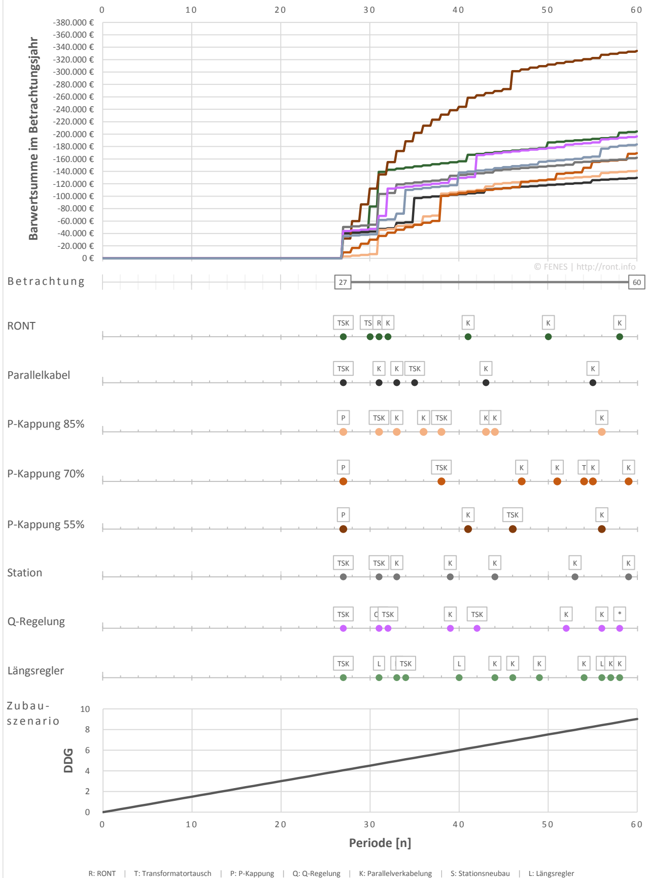
Abbildung 5: Zubau über 40 Jahre auf DDG_{norm} = 100\% , Stranganfang, i = 5\% | r = 1,5\% (KVE1)
