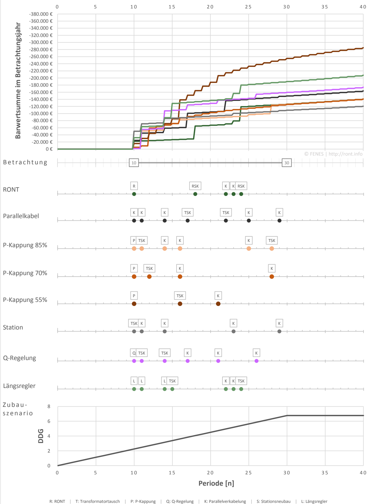
Abbildung 2: Zubau über 40 Jahre auf DDG_{norm} = 75\% , Strangende, i = 5\% | r = 1,5\% (KVE1)
