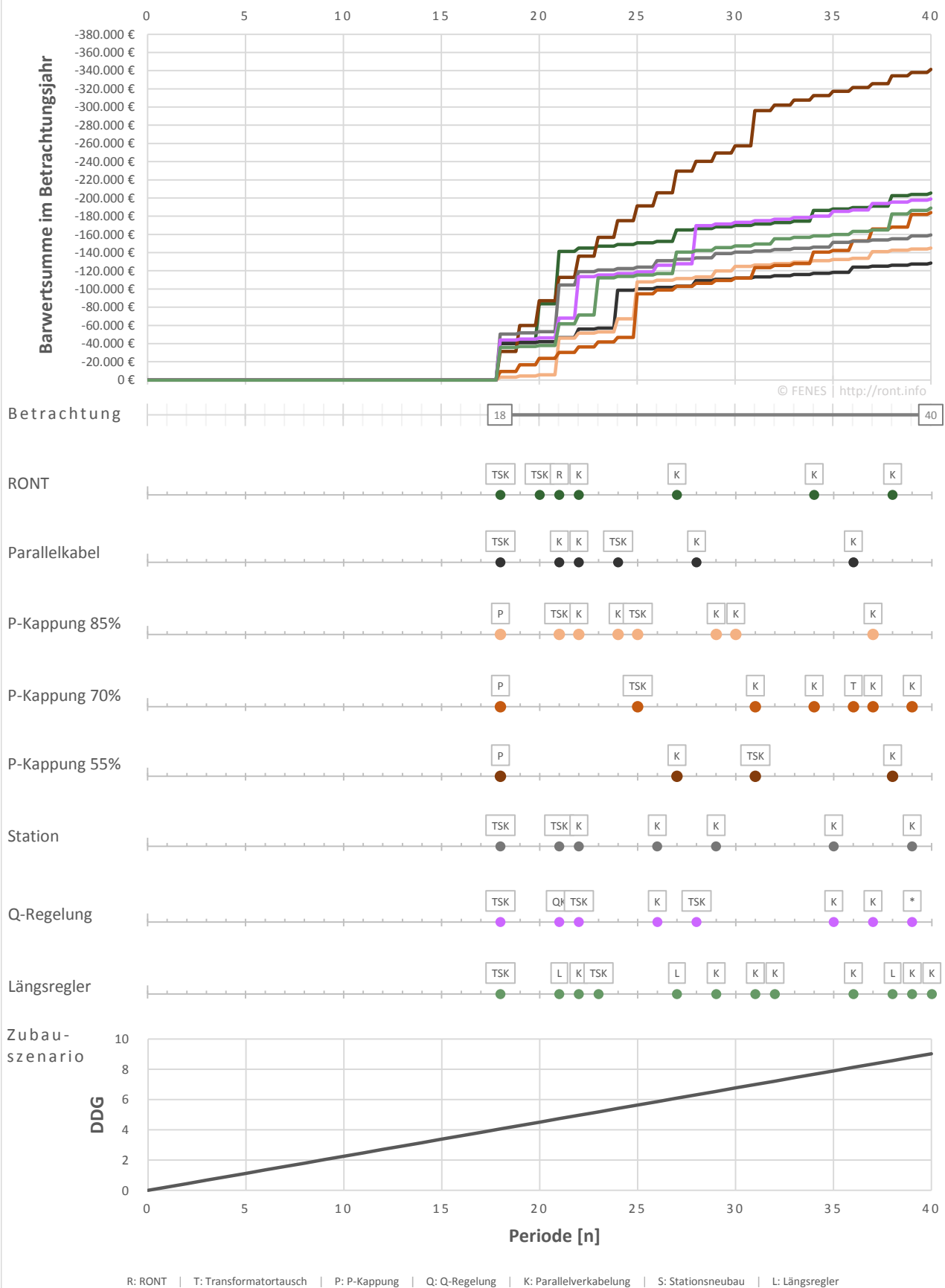
Abbildung 3: Zubau über 40 Jahre auf DDG_{norm} = 100\% , Stranganfang, i = 5\% | r = 1,5\% (KVE1)
