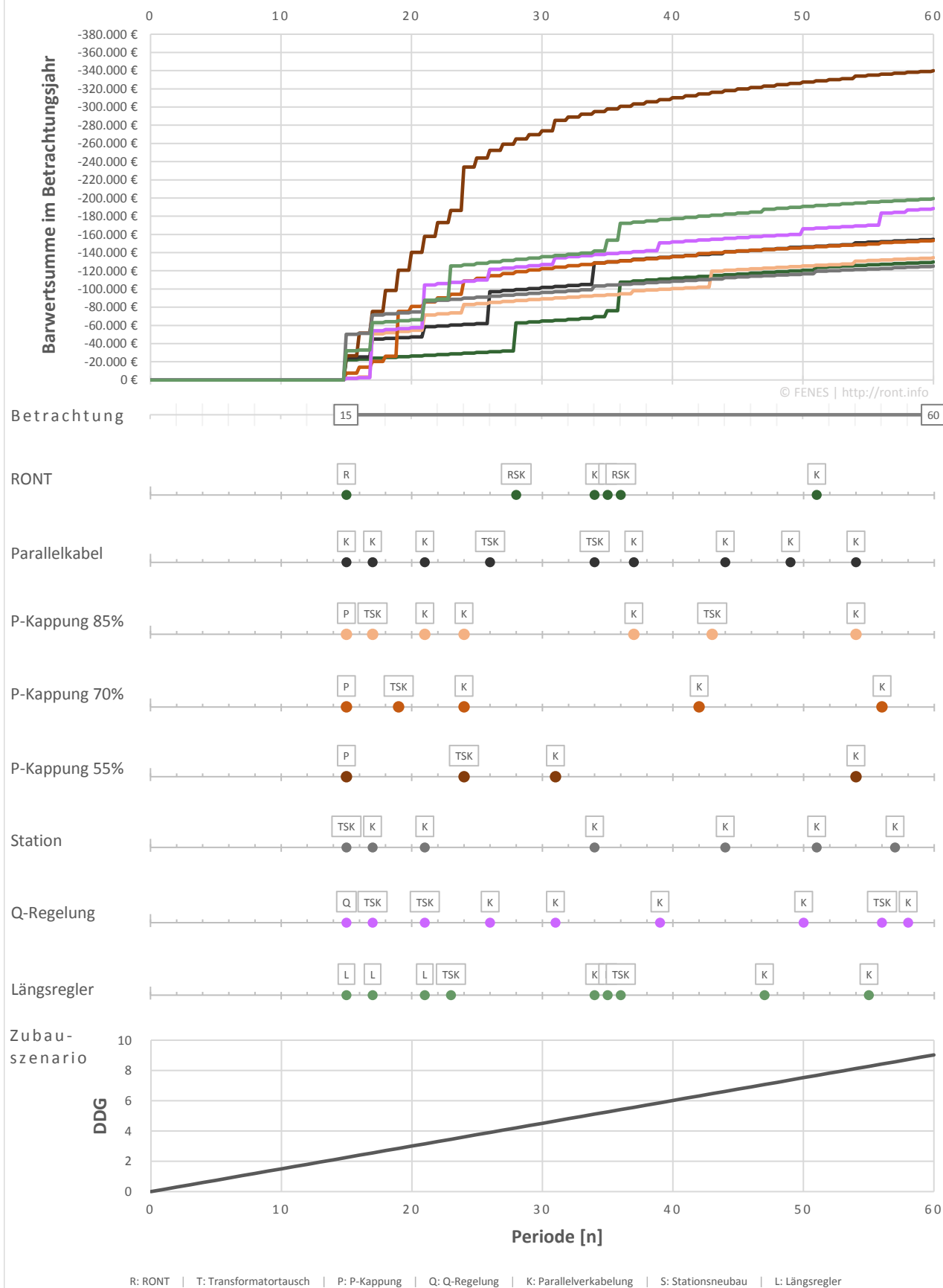
Abbildung 6: Zubau über 40 Jahre auf DDG_{norm} = 100\% , Strangende, i = 5\% | r = 1,5\% (KVE1)
