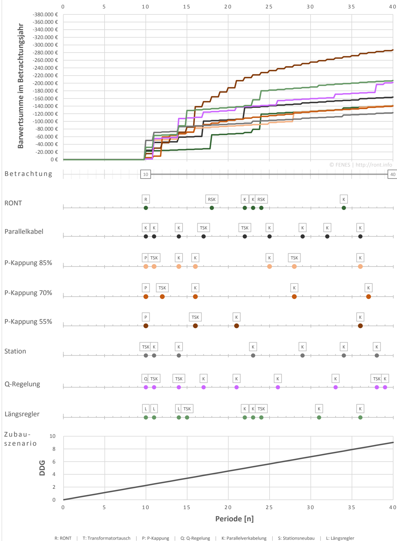
Abbildung 4: Zubau über 40 Jahre auf DDG_{norm} = 100\% , Strangende, i = 5\% | r = 1,5\% (KVE1)
